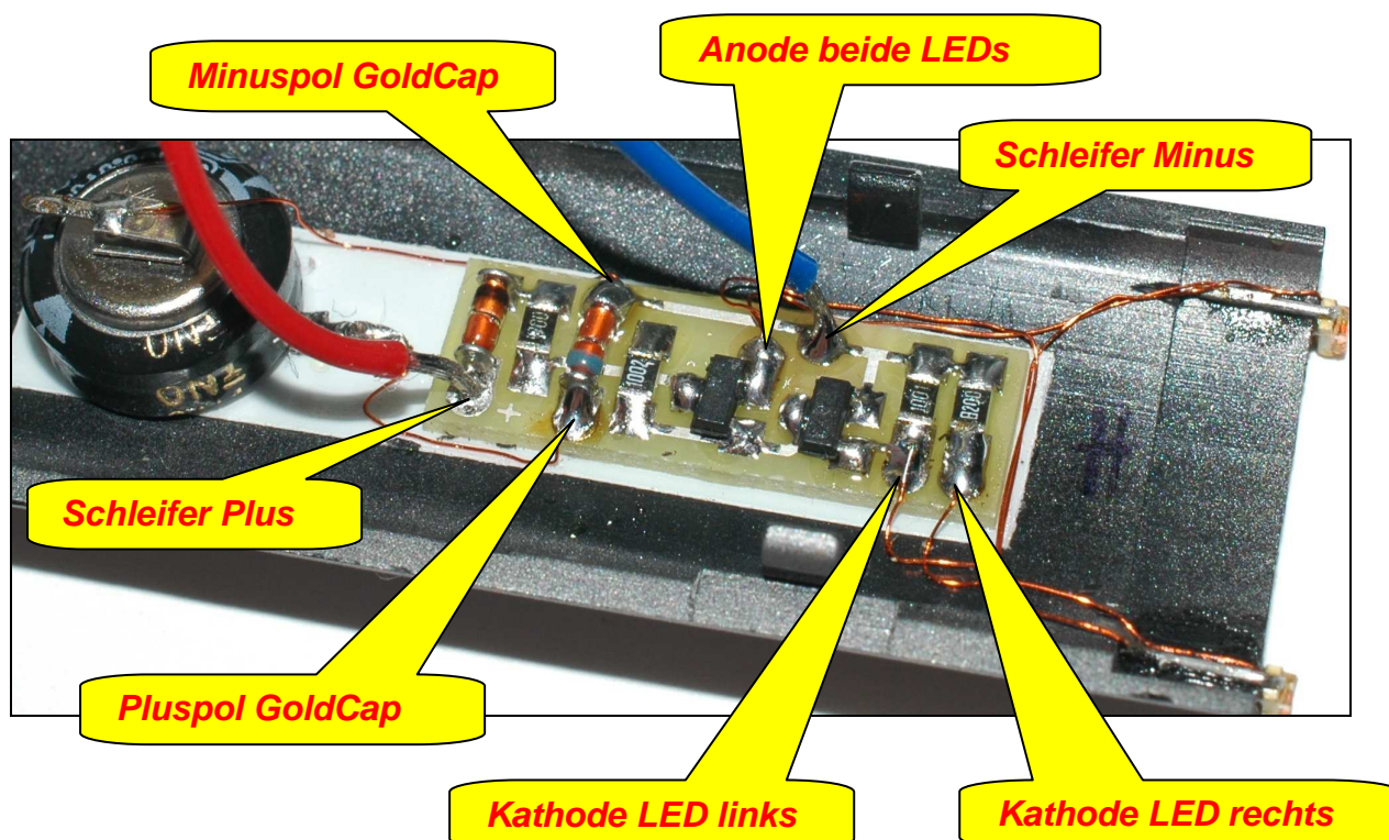
Bild 4.17: Verdrahtung im Detail
