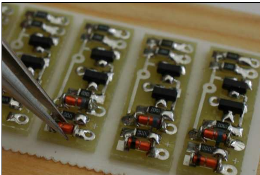
Bild 4.8: Platinen bei der Handbestückung
