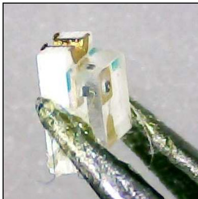
Bild 4.1: verwendete Chiplid
