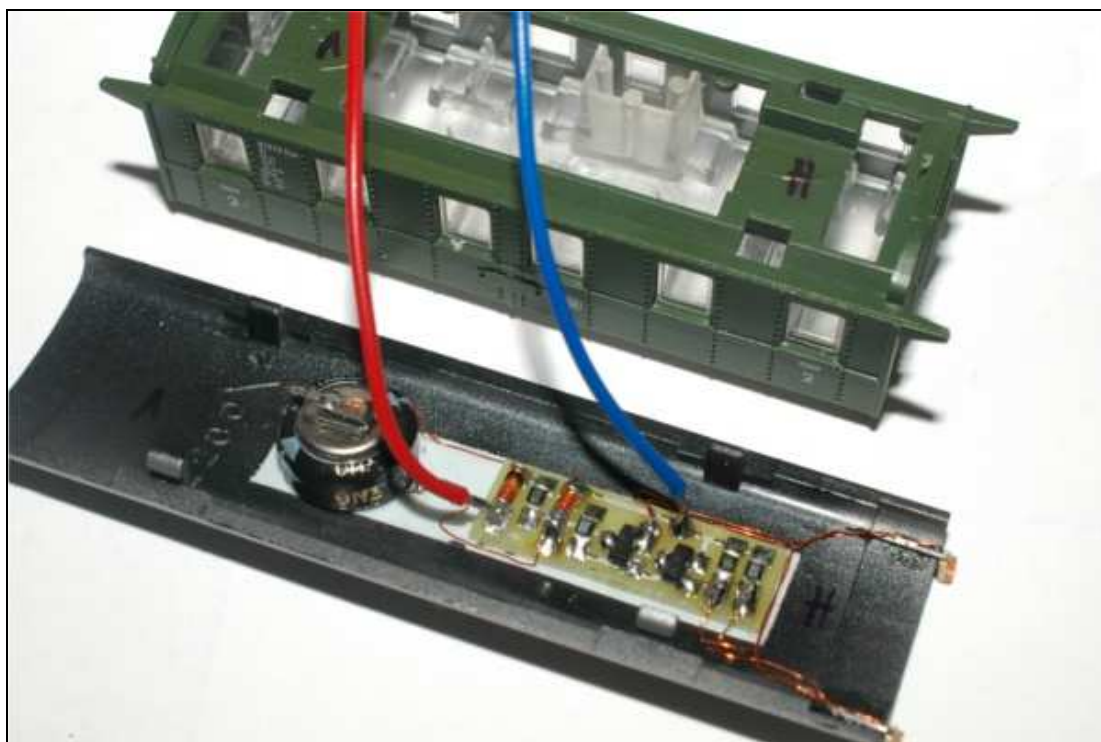
Bild 4.16: Einbau und Verdrahtung der Elektronik
