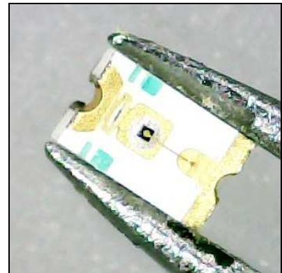
Bild 4.3: verwendete Chiplid
