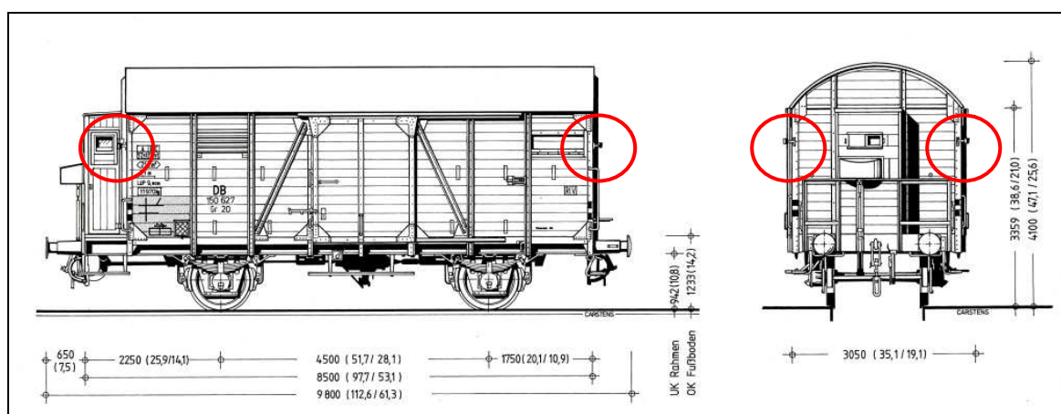
Bild 2.7: Signalstützen an einem G20 mBh
