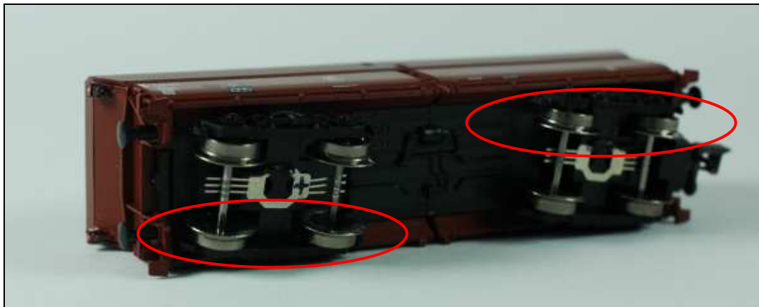
Bild 4.15: Drehgestellwagen mit Mayerhofer Schleifkontakten
