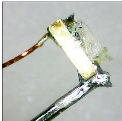
Bild 4.9: ChipLed mit montierten Anschlussdrähten
