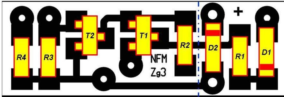
Bild 4.6: Bestückungsplan
