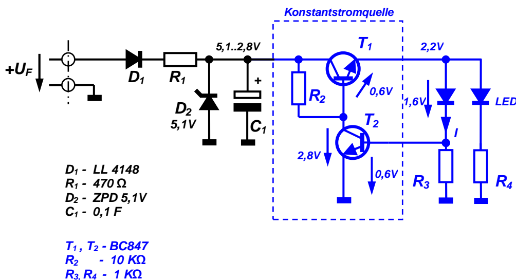
Bild 4.4: Schaltplan
