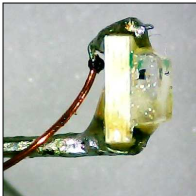
Bild 4.10: ChipLed mit montierten Anschlussdrähten
