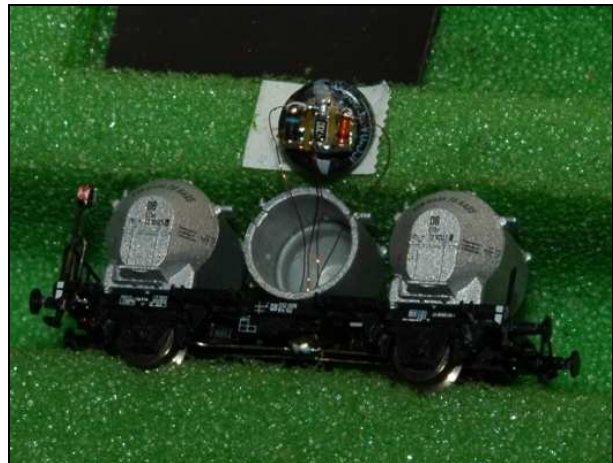
Bild 5.14: Montage der Konstantstromquelle Bild 5.15: Montage der Ladeschaltung
