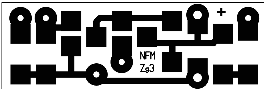
Bild 4.5: Schaltungslayout
